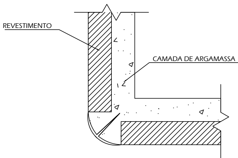
DETALHE DE FIXAÇÃO DA CANTONEIRA ESCALA 1/1
