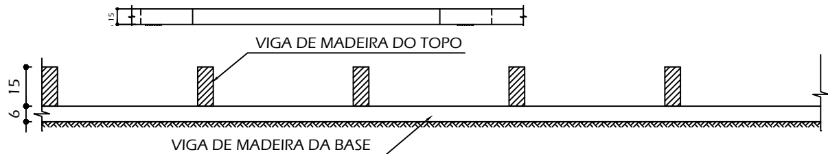
CORTE A-A
