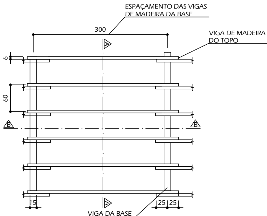
VISTA EM PLANTA
