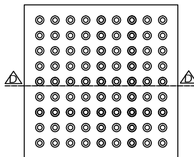
LADRILHO ALERTA 40x40 ESCALA 1/10
