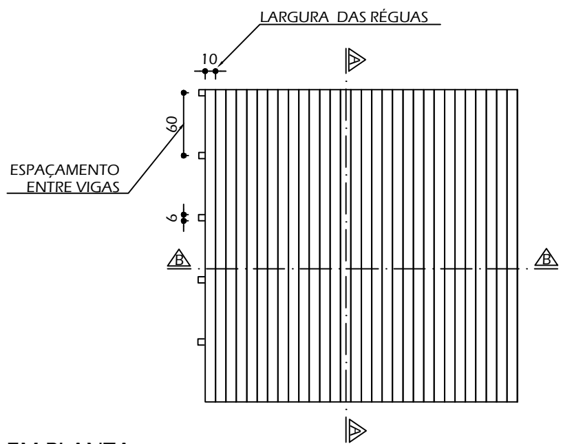
VISTA EM PLANTA ESCALA 1/50
