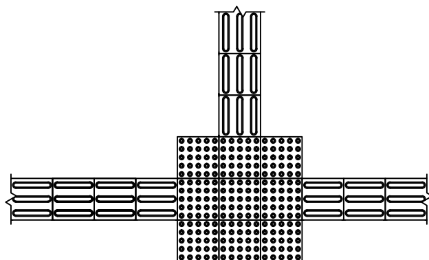
MUDANÇA DE DIREÇÃO/INTERSEÇÃO ESCALA 1/25
