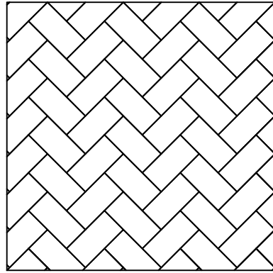
PADRÃO ESPINHA DE PEIXE ESCALA 1/20
