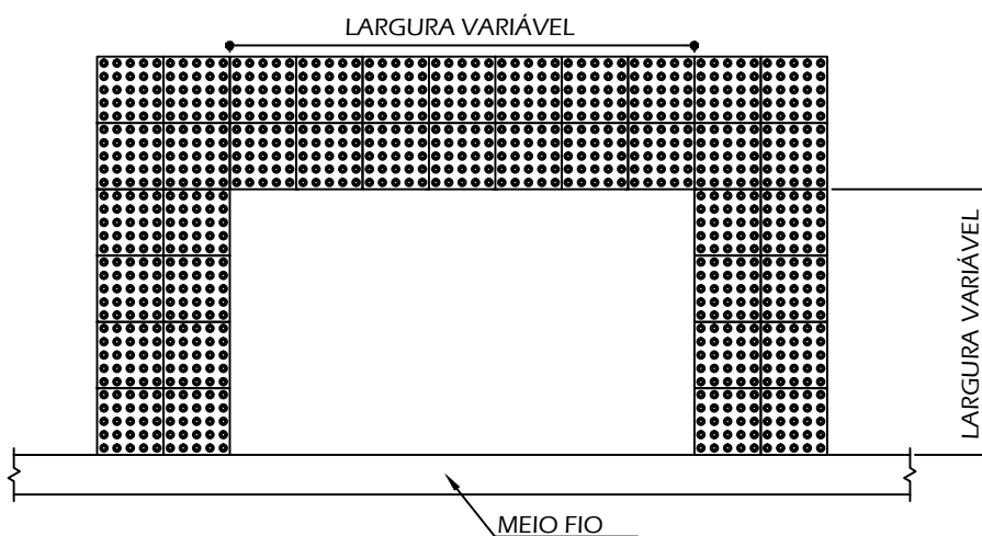
OBSTÁCULO/RAMPAMENTO PRÓXIMO À BORDA DO PASSEIO ESCALA 1/25
